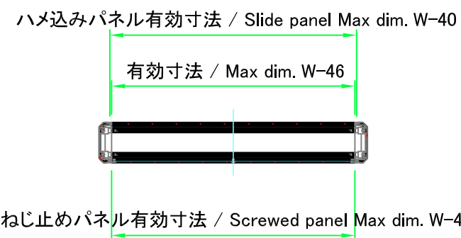
A-A ( 1 : 10 )
