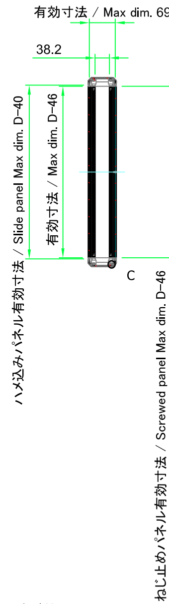
ナットレール / Nut rail
